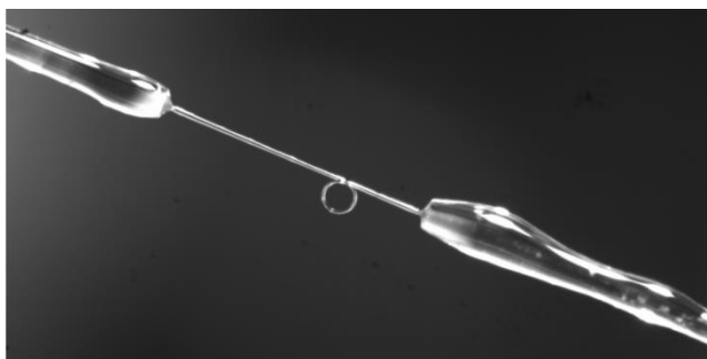
Obrázok: Optický vlákňový slučkový interferometer
